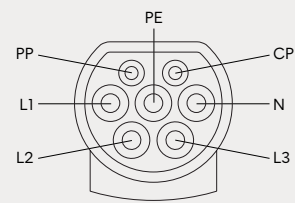
Ladestecker - Typ 2
