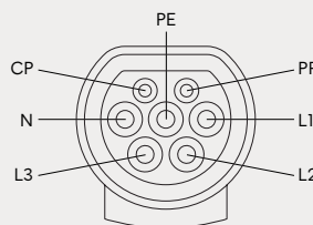
Fahrzeugstecker - Typ 2
